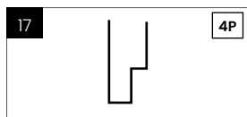
Czwarta przylga Nie dotyczy: • skrótu • głębokiego tloczenia Linii: • PERFECT • GLASS • GLASS VIEW • rozmiar "N" • drzwi dwuskrzydłowych • drzwi z dostawkami 4P
