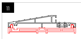
Poszerzenie podprogowe PCV 10 mm
