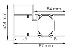
Profil ościeżnicy ALU/90
