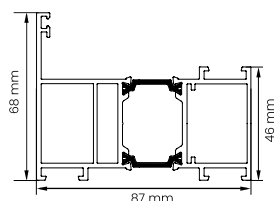
Profil naświetla
