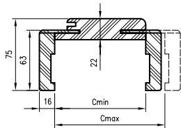
Przekrój OR/ORC z ką. T63
