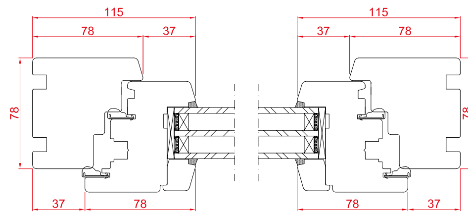
Przekrój A
