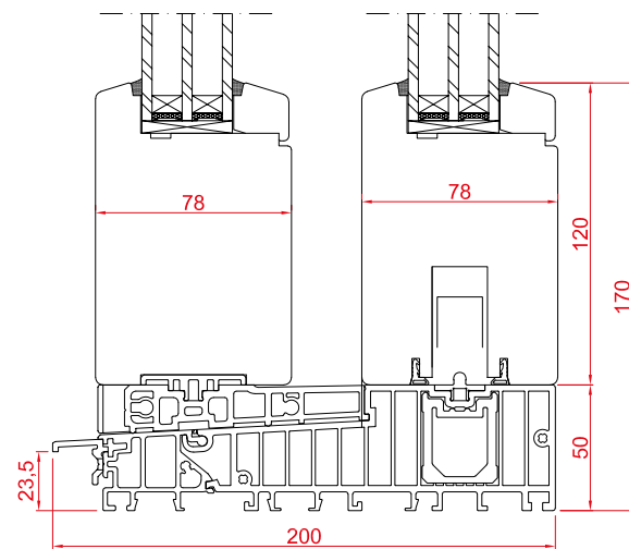
Przekrój D
