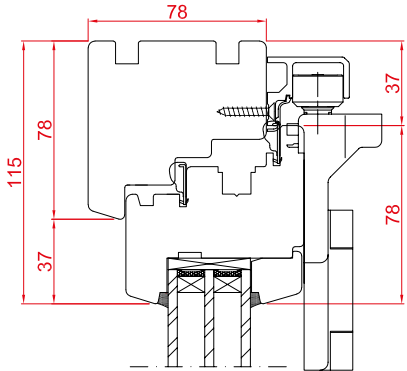
Przekrój B
