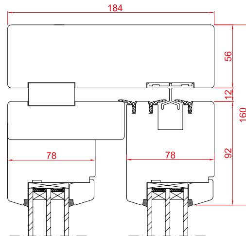
Przekrój B
