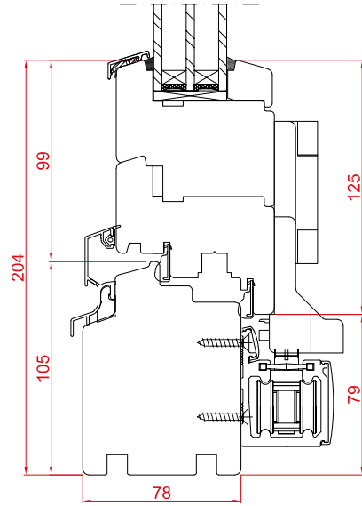
Przekrój D
