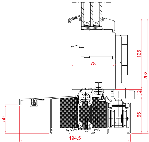
Przekrój D
